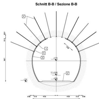
GALLERIE DI LINEA Ascavo = 65mq
