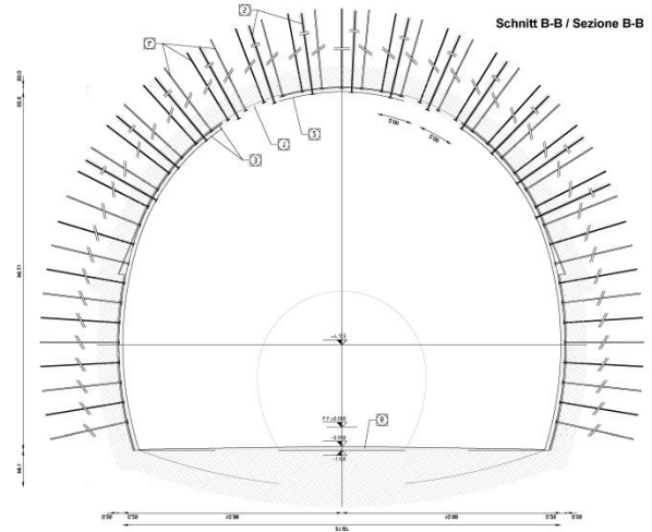
CAMERONE DI MONTAGGIO TBM E DI VENTILAZIONE Ascavo = 360mq
